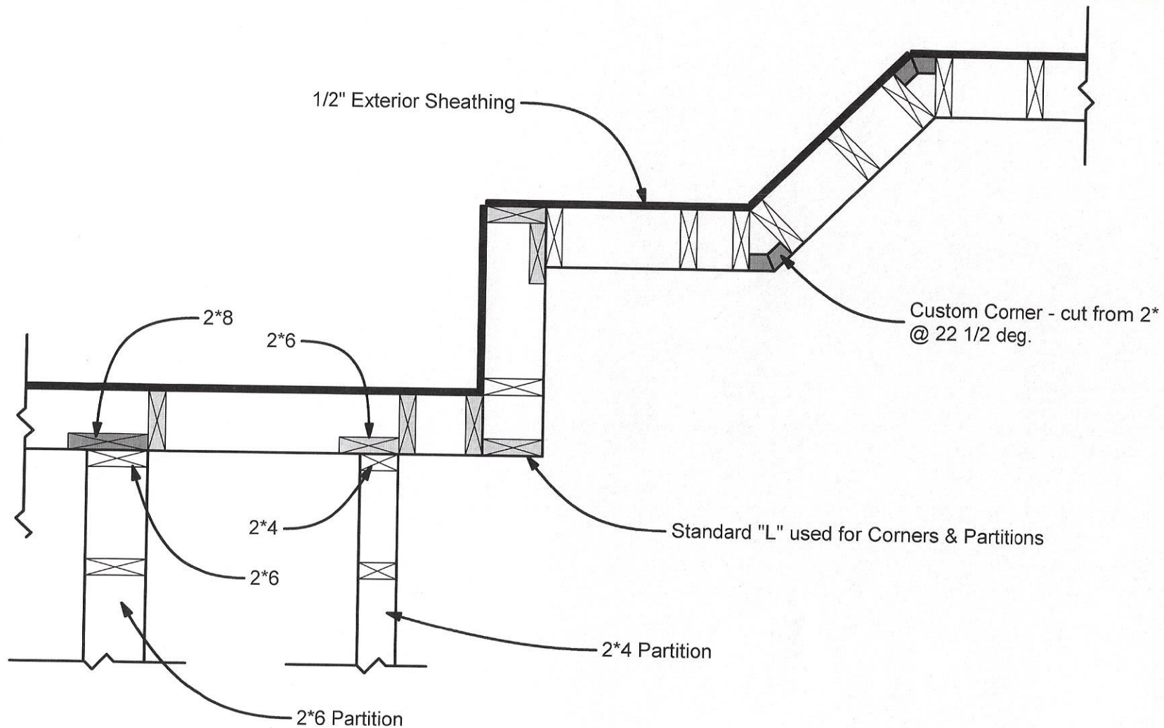
1 Stud Layout SCALE: 1" = 1'-0"
